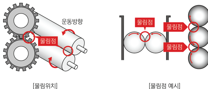
〈그림-21〉 물림점
