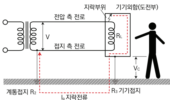
[나] 감전회로
